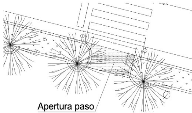
DETALLE APERTURA NOVO PASO
